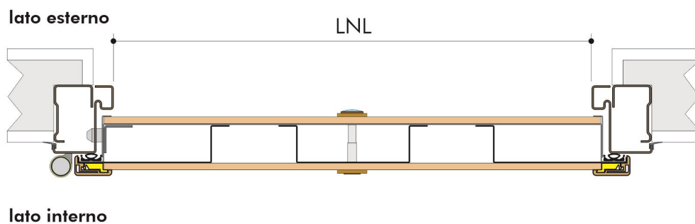
Schéma de renforcement vu de dessus
