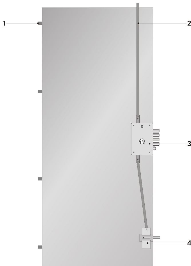
Schéma système de fermeture
